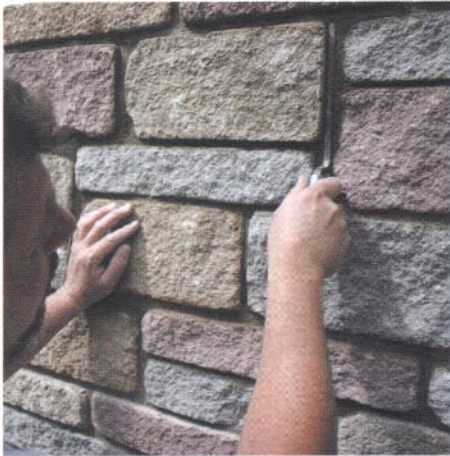
Die Fugen werden nicht bündig, sondern mindestens 5 mm tiefer als die Steinoberfläche ausgeformt.
